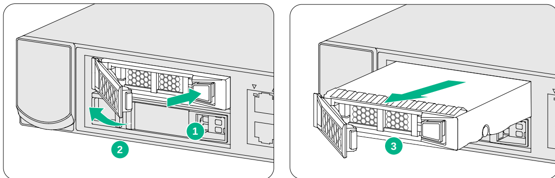
图4-3 更换硬盘
