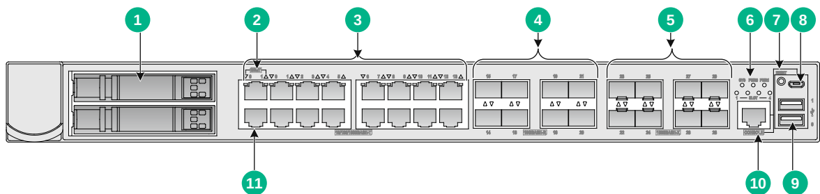
图A-1 设备前视图
