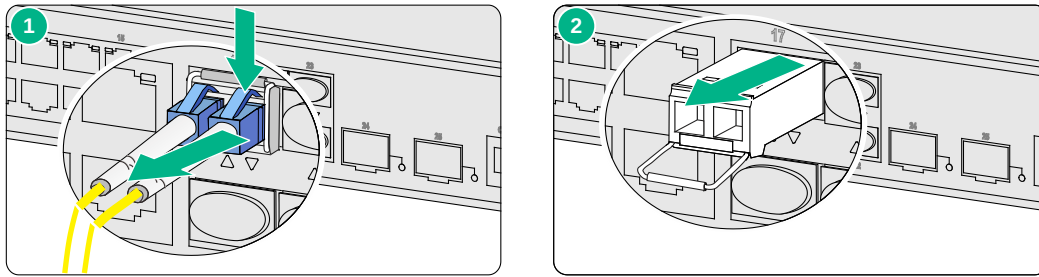
图4-5 拆卸光接口模块示意图
