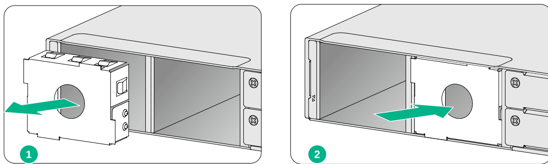
图2-11 拆卸电源假面板
