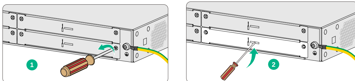
图2-13 拆卸假面板
