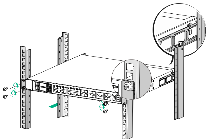
图2-7 安装设备到机柜（后挂耳正装）
