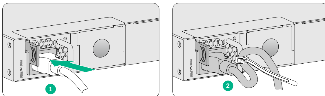
图2-19 连接交流电源线
