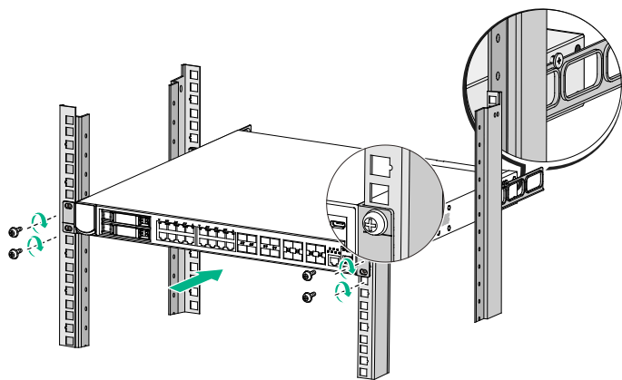
图2-8 安装设备到机柜（后挂耳反装）
