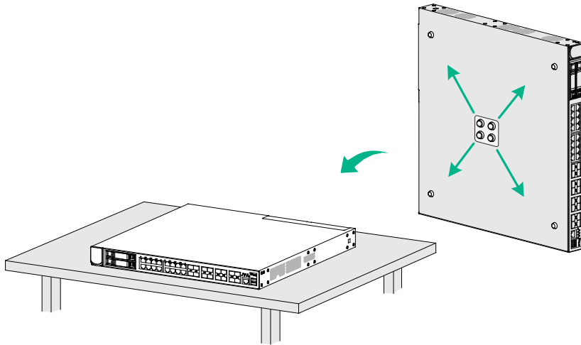
图2-2 工作台安装方式
