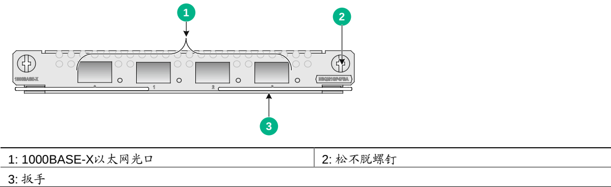
图A-5 NSQM1GP4FBA 接口模块正视图
