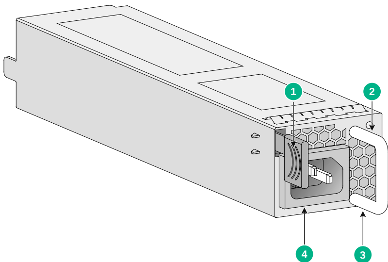
图A-7 PSR250-12A1 交流电源模块外观
