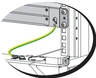
图2-10 连接到机柜接地
