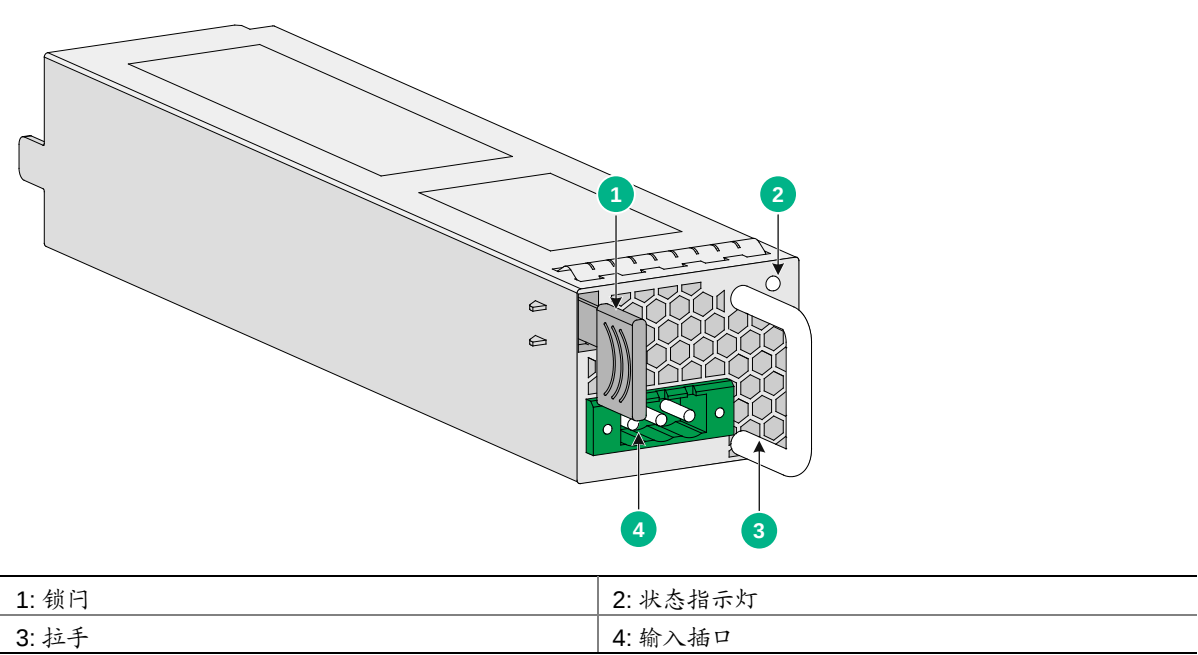
图A-8 PSR450-12D 直流电源模块外观
