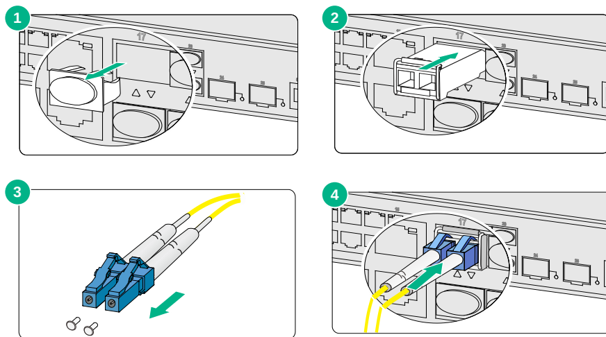
图2-18 安装及连接光模块
