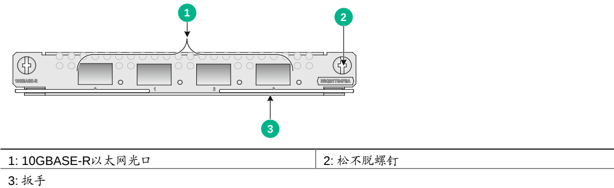
图A-4 NSQM1TG4FBA 接口模块正视图
