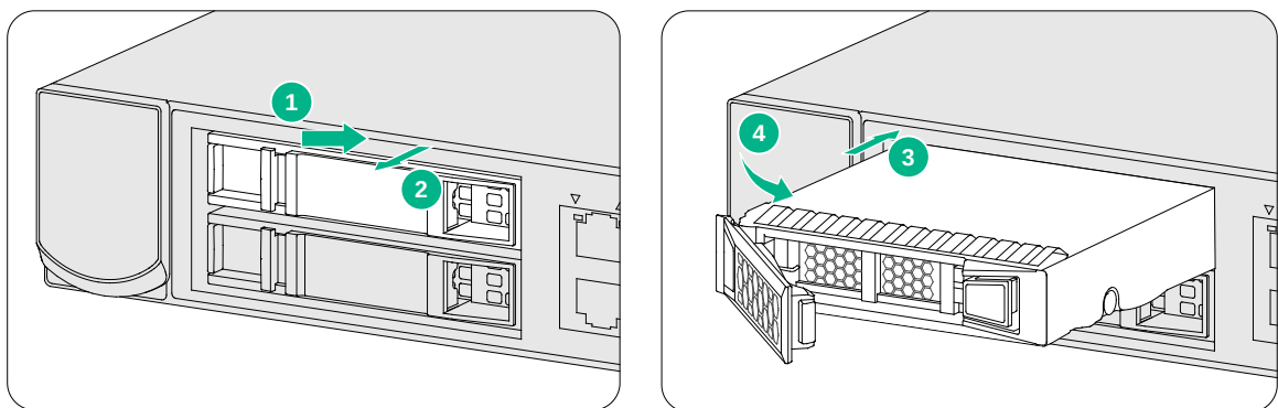
图2-15 安装硬盘
