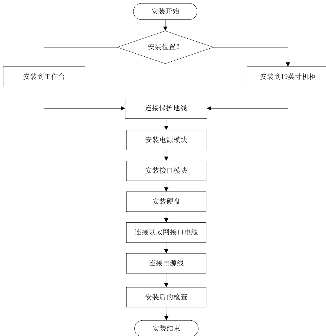
图2-1 设备安装流程示意图
