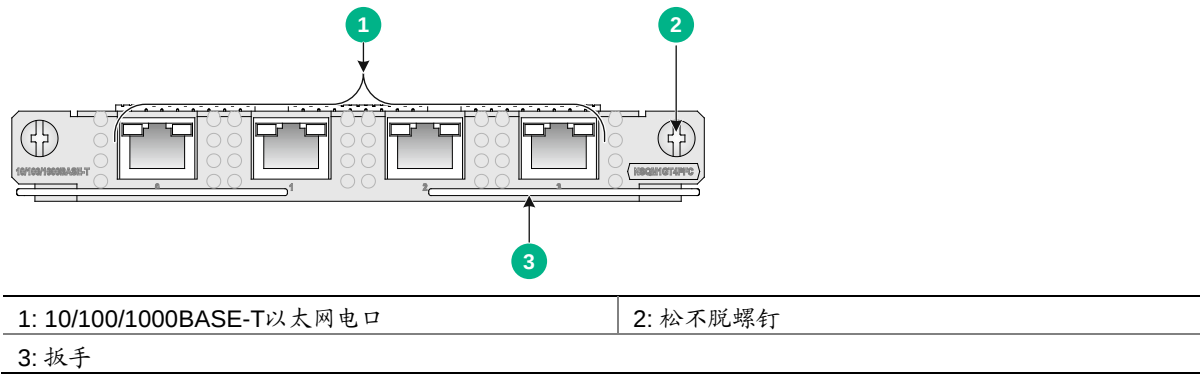
图A-3 NSQM1GT4PFC 接口模块正视图
