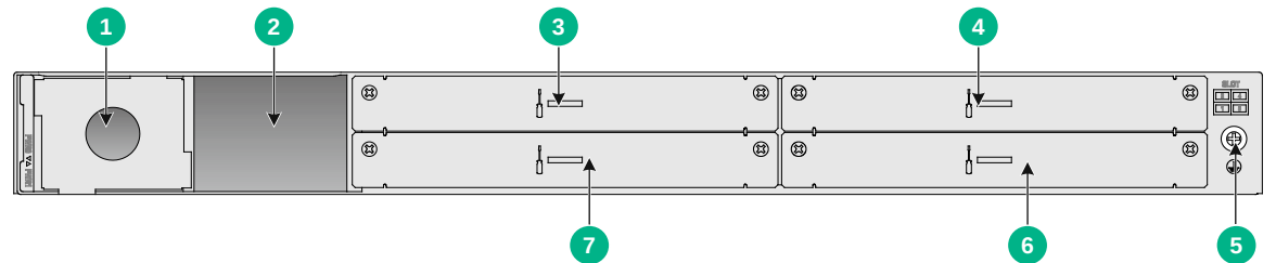
图A-2 设备后视图
