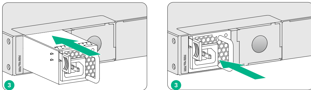
图2-12 安装电源模块
