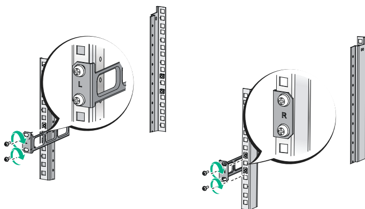
图2-5 安装后挂耳（后挂耳正装）
