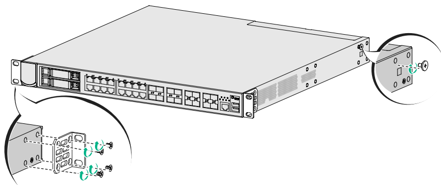
图2-4 安装前挂耳和承重螺钉
