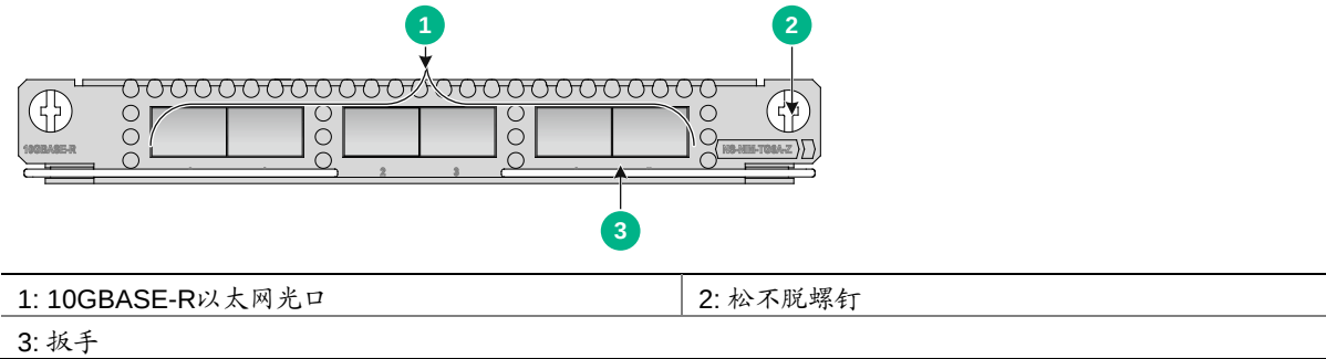
图A-6 NS-NIM-TG6A-Z 接口模块正视图
