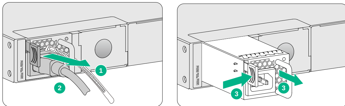
图4-1 拆卸电源模块
