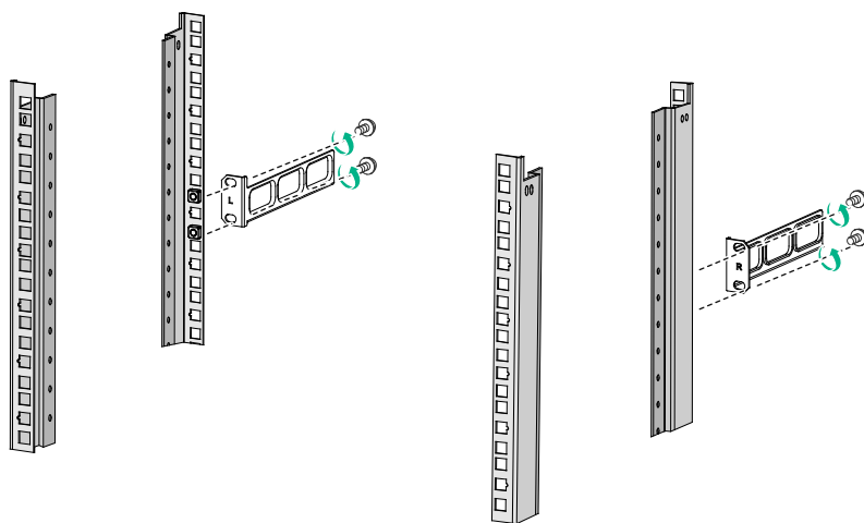
图2-6 安装后挂耳（后挂耳反装）
