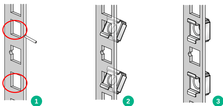
图2-3 安装浮动螺母
