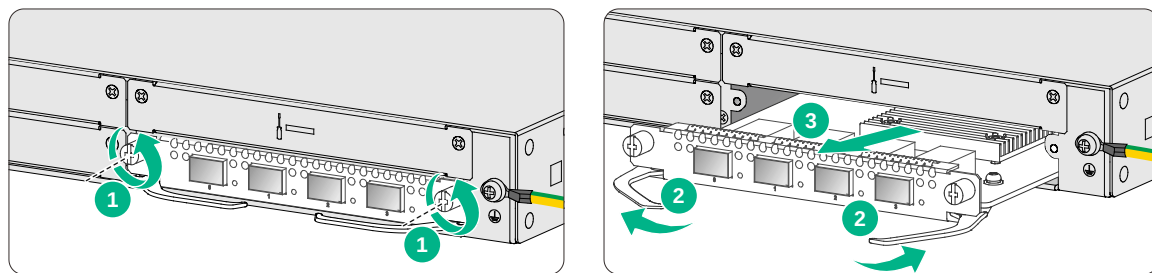
图4-2 拆卸接口模块
