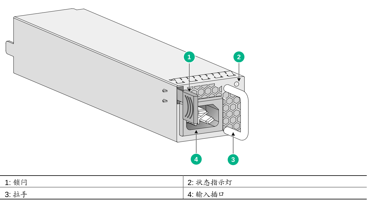
图A-9 PSR450-12AHD 高压直流电源模块外观
